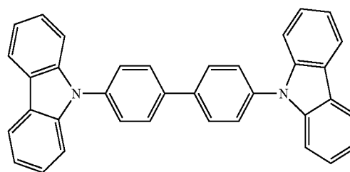
CBP
