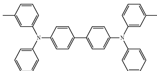
TPD
