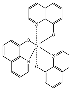
Alq 3
